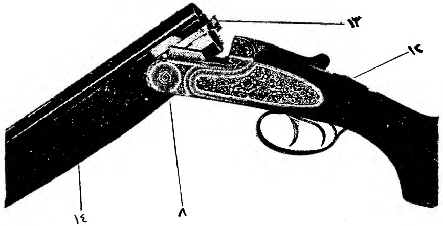
جفت « بماسورتين » فوق بعضها في حالة الفتح ( لاحظ النازع رقم ١٣ )
